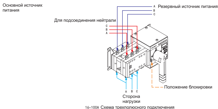
16-100А Схема трехполюсного подключения
