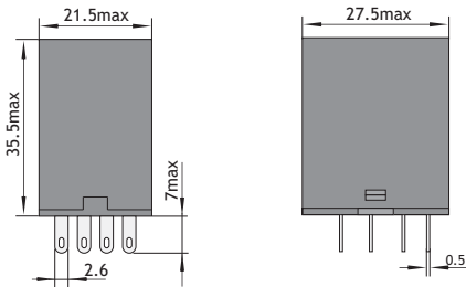
JZX-22F(D)/4-03
