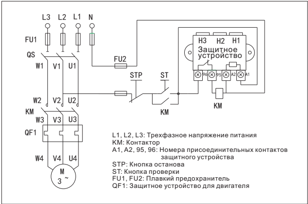
7.1 На рис. 2 показана схема соединений цепи управления для напряжения 220 и 230 В.
