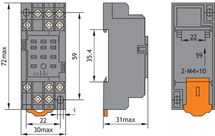
72×30×31 (мм)
