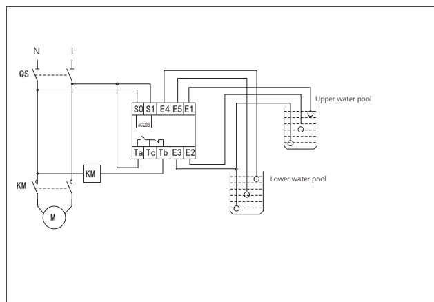
Для NJYW1-BL1, NJYW1-BL2 напряжение питания 220В
