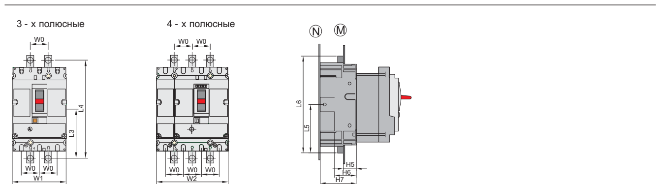
Расположение монтажных панелей
