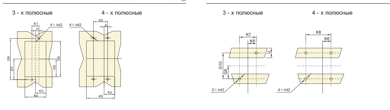
Разметка шин
