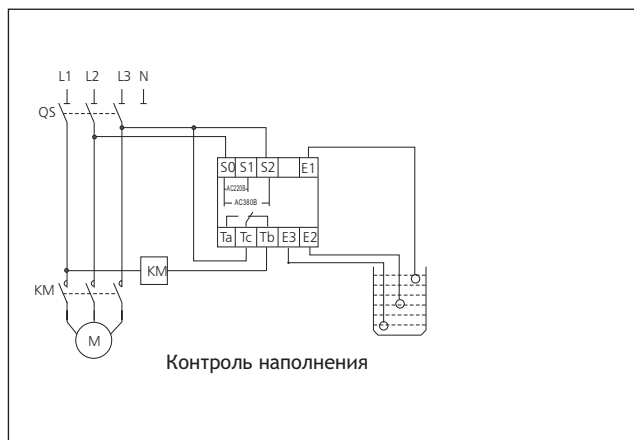
Для NJYW1-NL1, NJYW1-NL2 напряжение питания 220/380В
