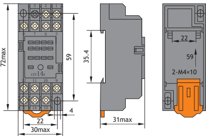
72×30×31 (мм)
