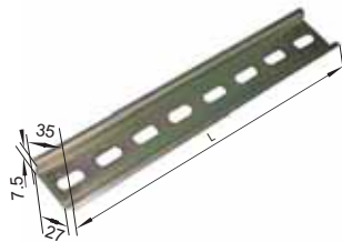
Размеры монтажной рейки
