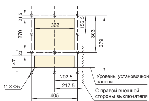
Положения отверстия на панели
