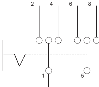
NZK1-32/2
