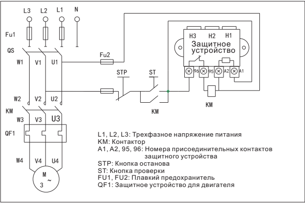
7.2 На рис. 3 показана схема соединений цепи управления для напряжения 380 и 400 В.
