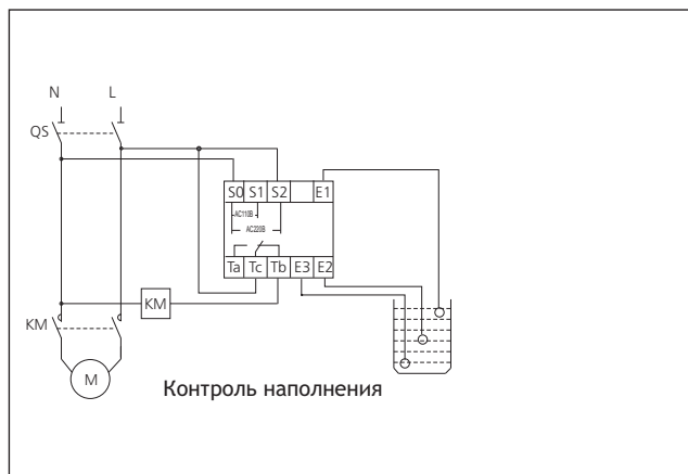
Для NJYW1-NL1, NJYW1-NL2 напряжение питания 110V/220В
