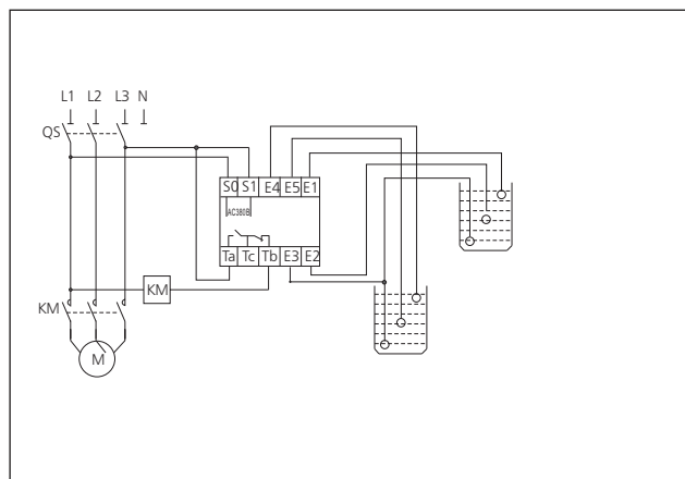
Для NJYW1-BL1, NJYW1-BL2 напряжение питания 380В
