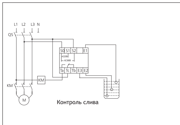
Для NJYW1-NL1, NJYW1-NL2 напряжение питания 220V/380В
